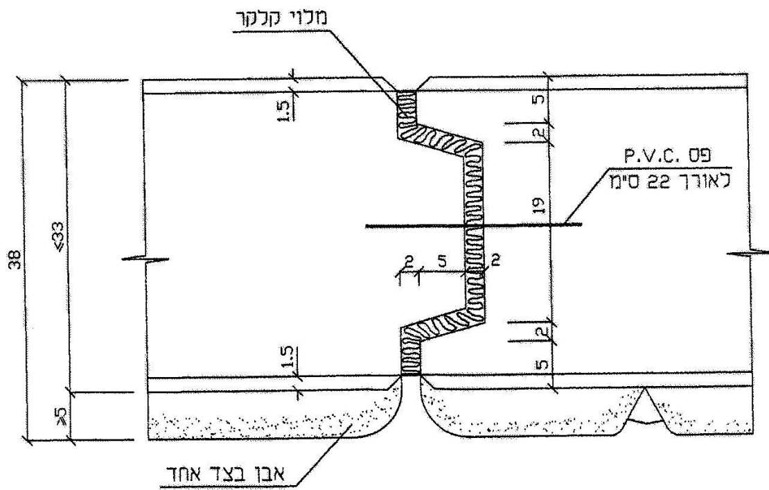
תפר התפשטות 1:5
