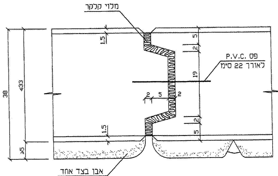
תפר התפשטות 1:5
